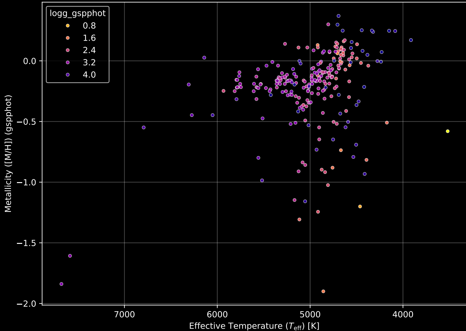
APOGEE DR17 Field: [270-12] Stellar Population Parameters (n= 253)
